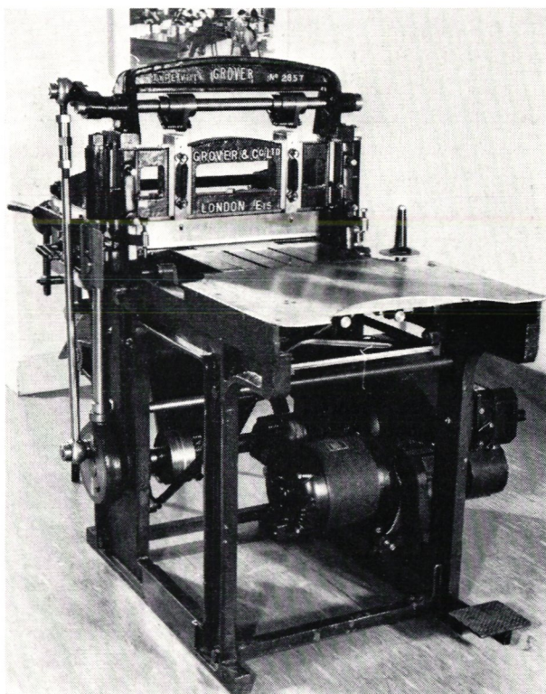
Perforeringsmaskin för frimärken av Grovers tillverkning, London.
