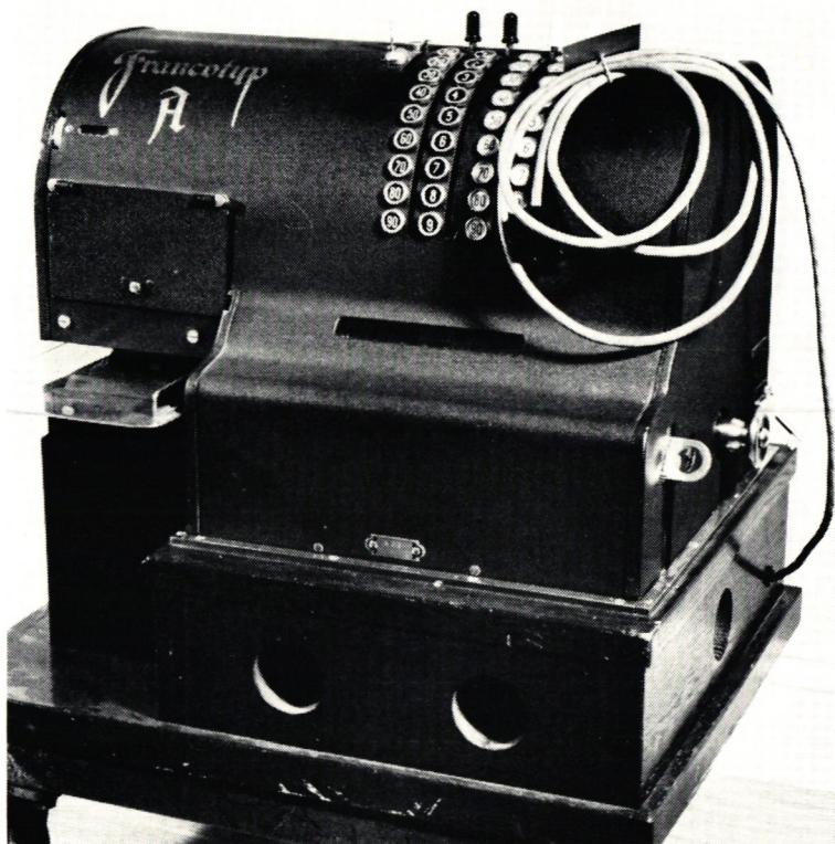
Frankostämpplingsmaskin av märket »Frankotyp A». Gåva av AB Carl Lamm.
