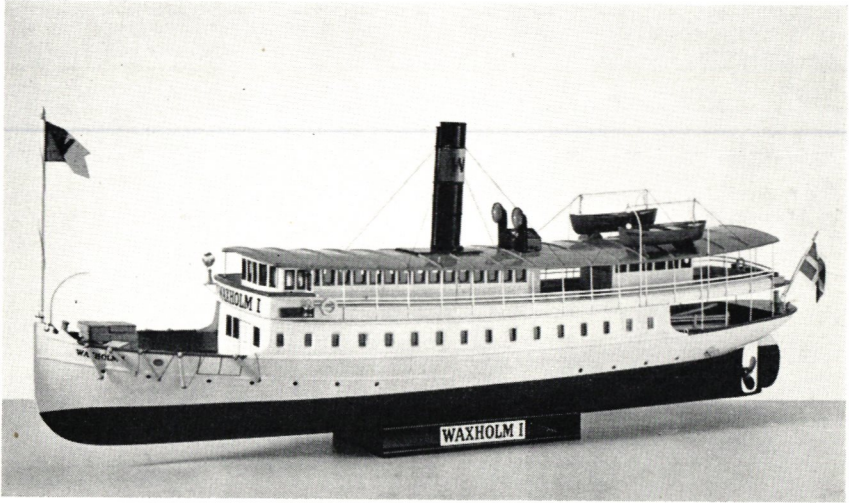
Waxholm I modell i skalan 1/62 byggd av tekn. stud. Ingmar Lind efter en konstruktionsritning av ingenjör Sigurd Isacson.
