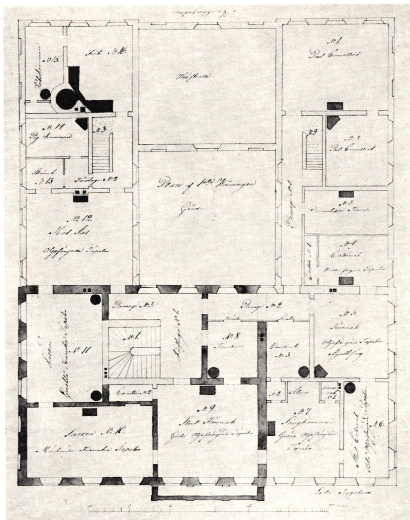
Ritning till Stockholms posthus ombyggnad på 1820-talet. Våningen 1 trappa upp. Efter original i Generalpoststyrelsen.
