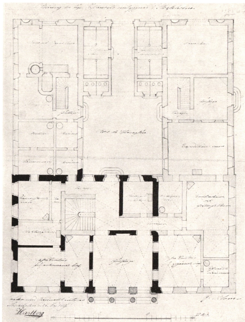
Ritning till Stockholms posthus ombyggnad på 1820-talet. Bottenvåningen. Efter original i Generalpoststyrelsen.
